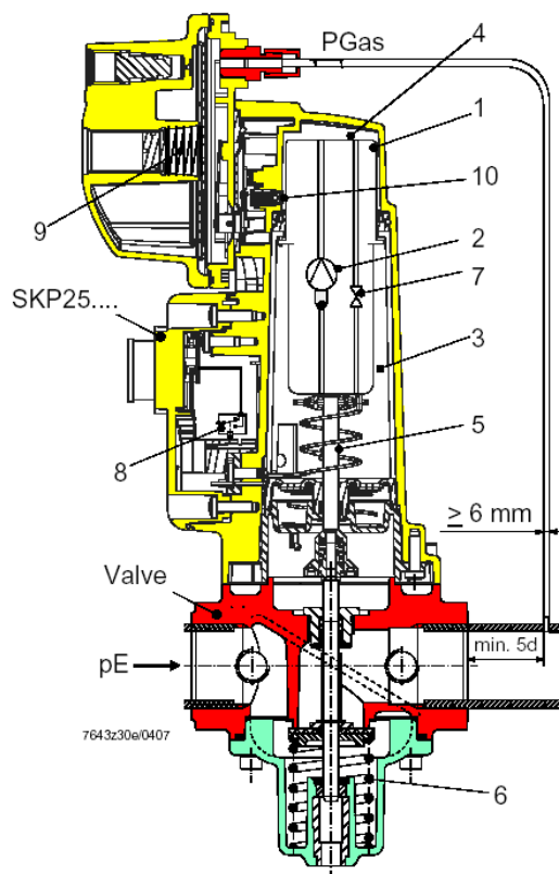
アクチュエータ内部断面図
