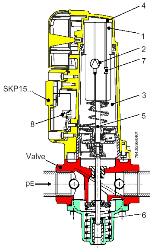
アクチュエータ内部断面図
