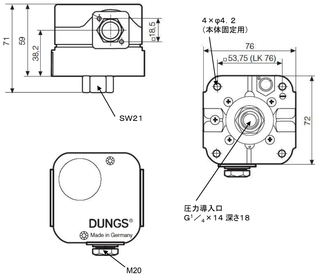
外形寸法図
