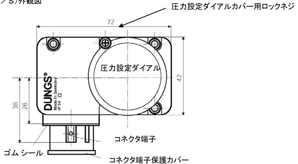
ガス圧高 (GW A6 / S) 外観図
