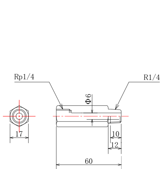
導圧管アダプタ 材質: C3604
