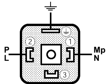
端子 配線図
